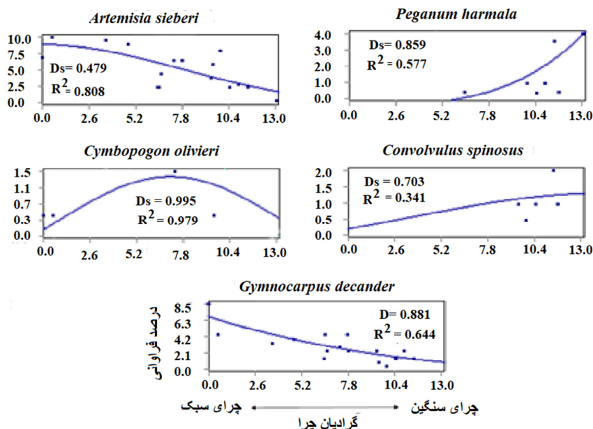
شکل ۵: منحنی پاسخ گونه‌های معرف به چرا در منطقه مطالعاتی حاجی آباد هرمزگان همراه با شاخص پذیرش (Ds) و ضریب تبیین (R 2 ) هر کدام از آن‌ها: محور افقی نشان‌دهنده گرادیان چرایی (از سمت چپ به سمت راست افزایش فشار چرا) و محور عمودی نشان‌دهنده فراوانی گونه در یک فشار چرایی معین می‌باشد.
